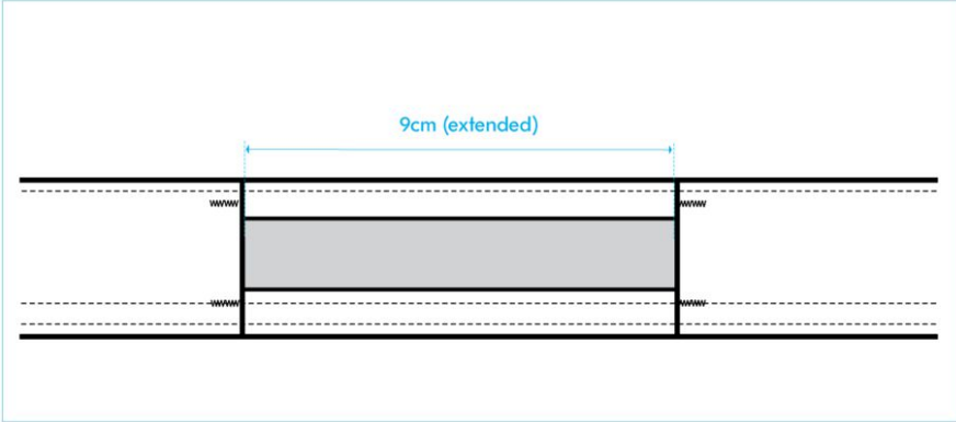
BACK WAISTBAND
